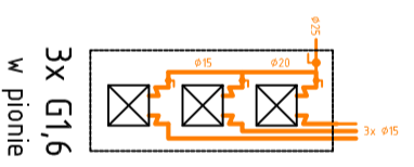
Schemat szafki gazomierzowej
